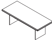
СТОЛ ПЕРЕГОВОРОВ (OTM220) Ш: 220 / Г: 95 / В: 75
