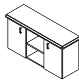
ГРЕДЕНЦИЯ (OTM203) Ш: 143 / Г: 45 / В: 74,4
